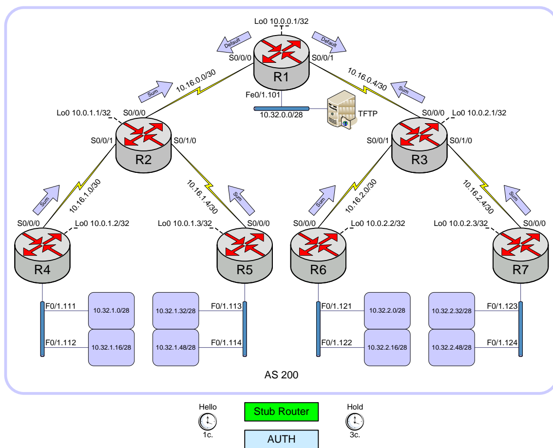
Рисунок 10 – Структурная схема стенда лабораторной работы №10
